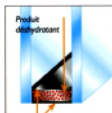
Double joint d'étanchéité
